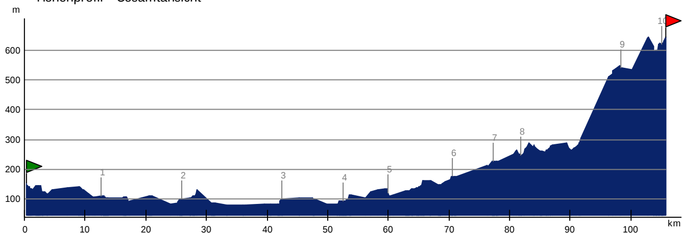
Höhenprofil - Gesamtansicht
